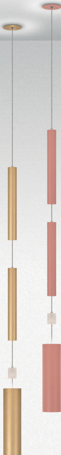
PENDENTE FLOAT 2096 Porta lâmpada: 2 x GU10 MR11 Difusor: Acrílico fosco Luminária: Ø 51 x \Phi 180 mm Módulos ajustáveis em metal e acrílico fosco Base de teto Full Contact: Ø 55 x 3 mm Cabo de alimentação: \Phi 2 m (regulável)
